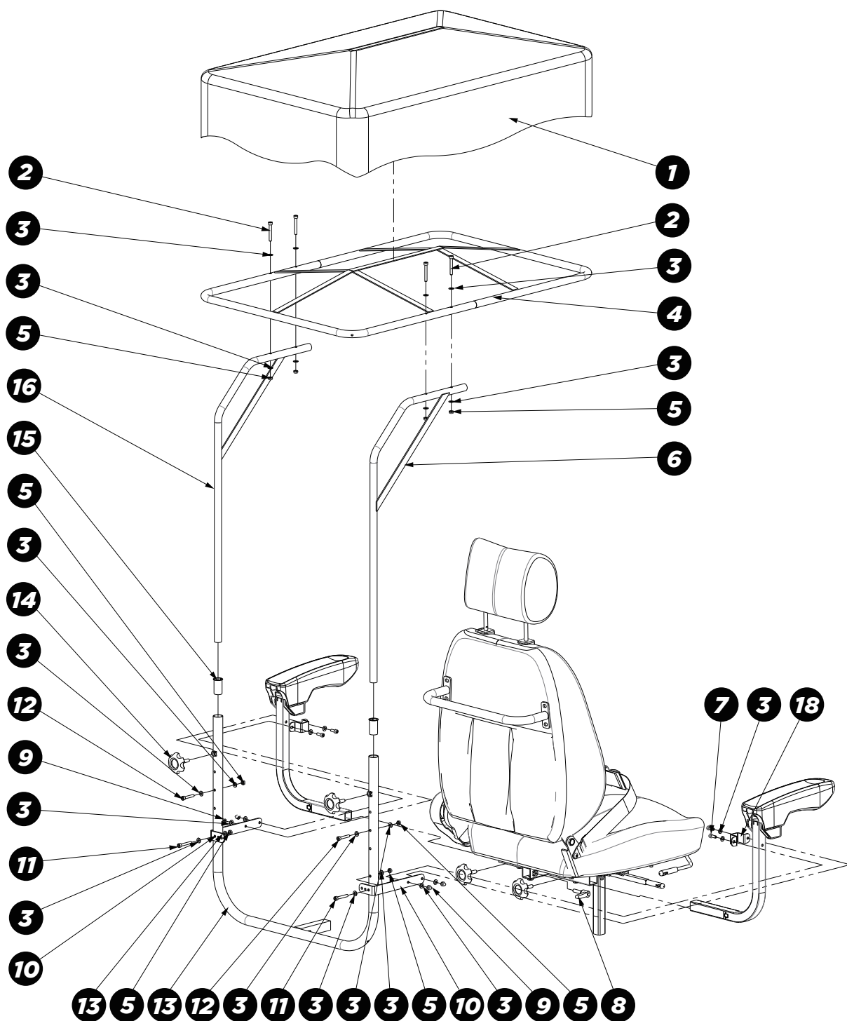
遮 陽 棚 組 合 圖
